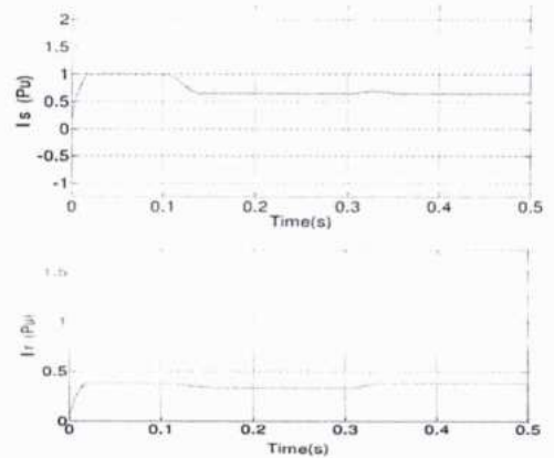
(d) Stator and rotor currents.
