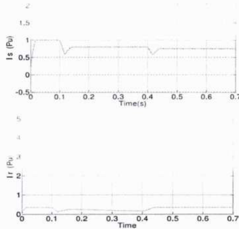
(d) Stator and rotor currents.
